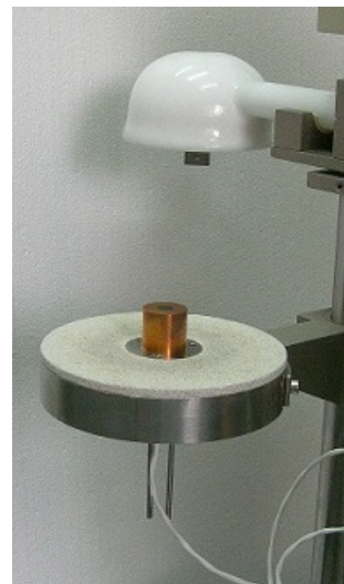
Gardon radiometer
